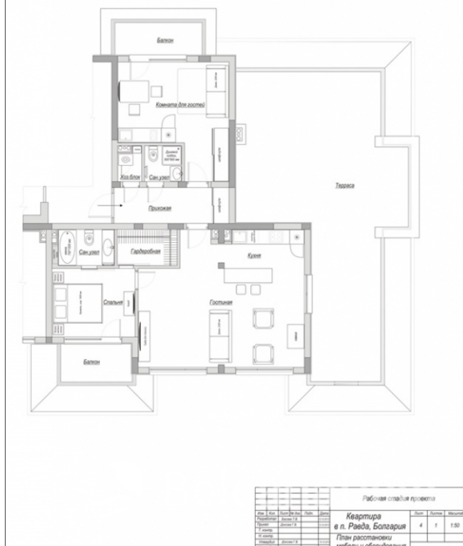
План расстановки мебели и оборудования М 1:50
